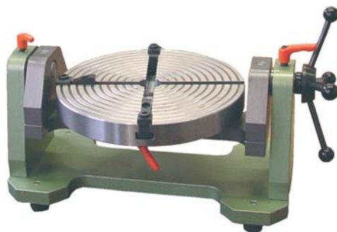
Поворотный стол с зажимным диском \varnothing 250 мм
