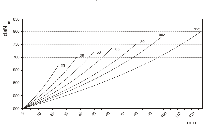
Wskaźnik siły / skoku • Force / stroke ratio
