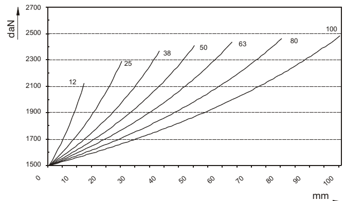
Wskaźnik siły / skoku • Force / stroke ratio
