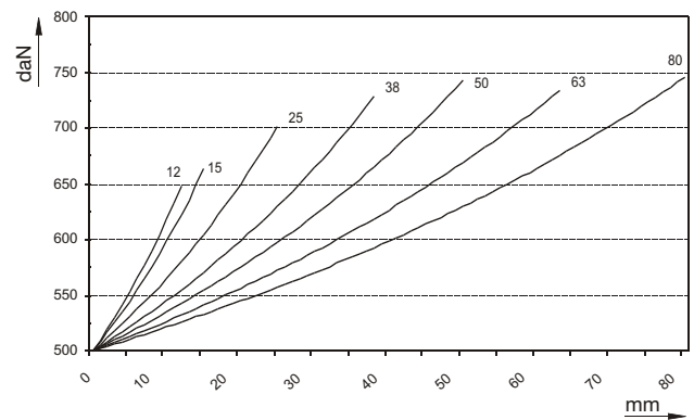
Wskaźnik siły / skoku • Force / stroke ratio
