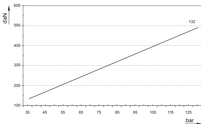
Wskaźnik siły / ciśnienia • Force / pressure ratio
