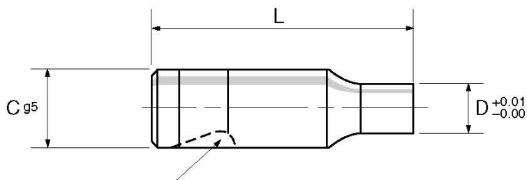
Heavy Duty Ball Seat – Wybranie pod kulkę do wysokich obciążeń
