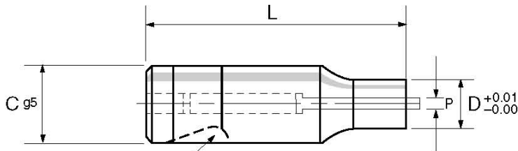
Light Duty Ball Seat – Wybranie pod kulkę do niskich obciążeń
