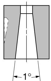
TAPER RECESS Wybieg stożkowy
