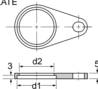
RETAINING – PŁYTKA PODTRZYMUJ CA PLATE
